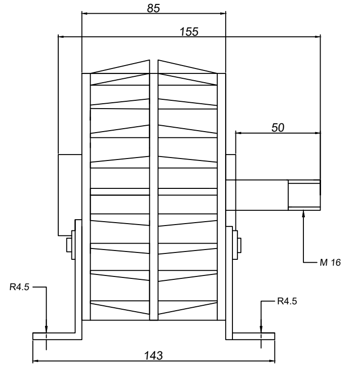
500W AYAKLI ALTERNATÖR
