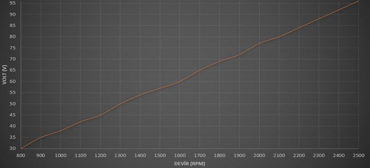
G-500 24V Alternatör Devir-Volt Grafiği
